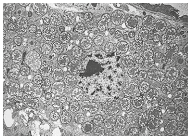
Buchnera aphidicola
